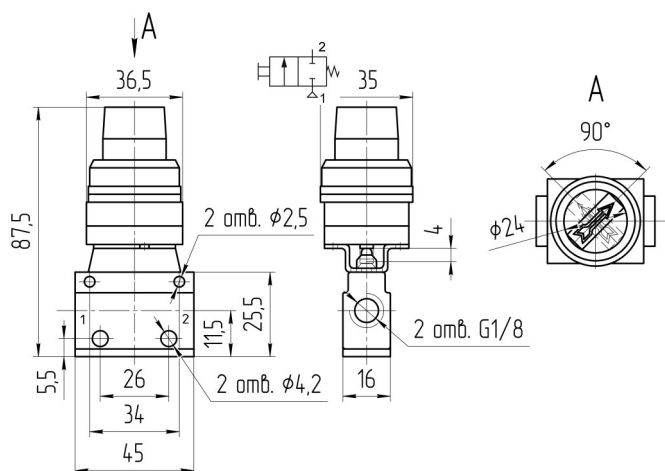
ПНЕВМОРАСПРЕДЕЛИТЕЛЬ ДВ76-221
