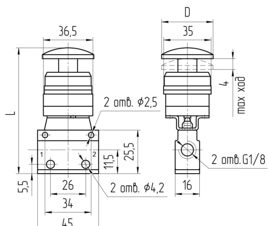
ПНЕВМОРАСПРЕДЕЛИТЕЛЬ ЕВ76(ТВ76)-221
